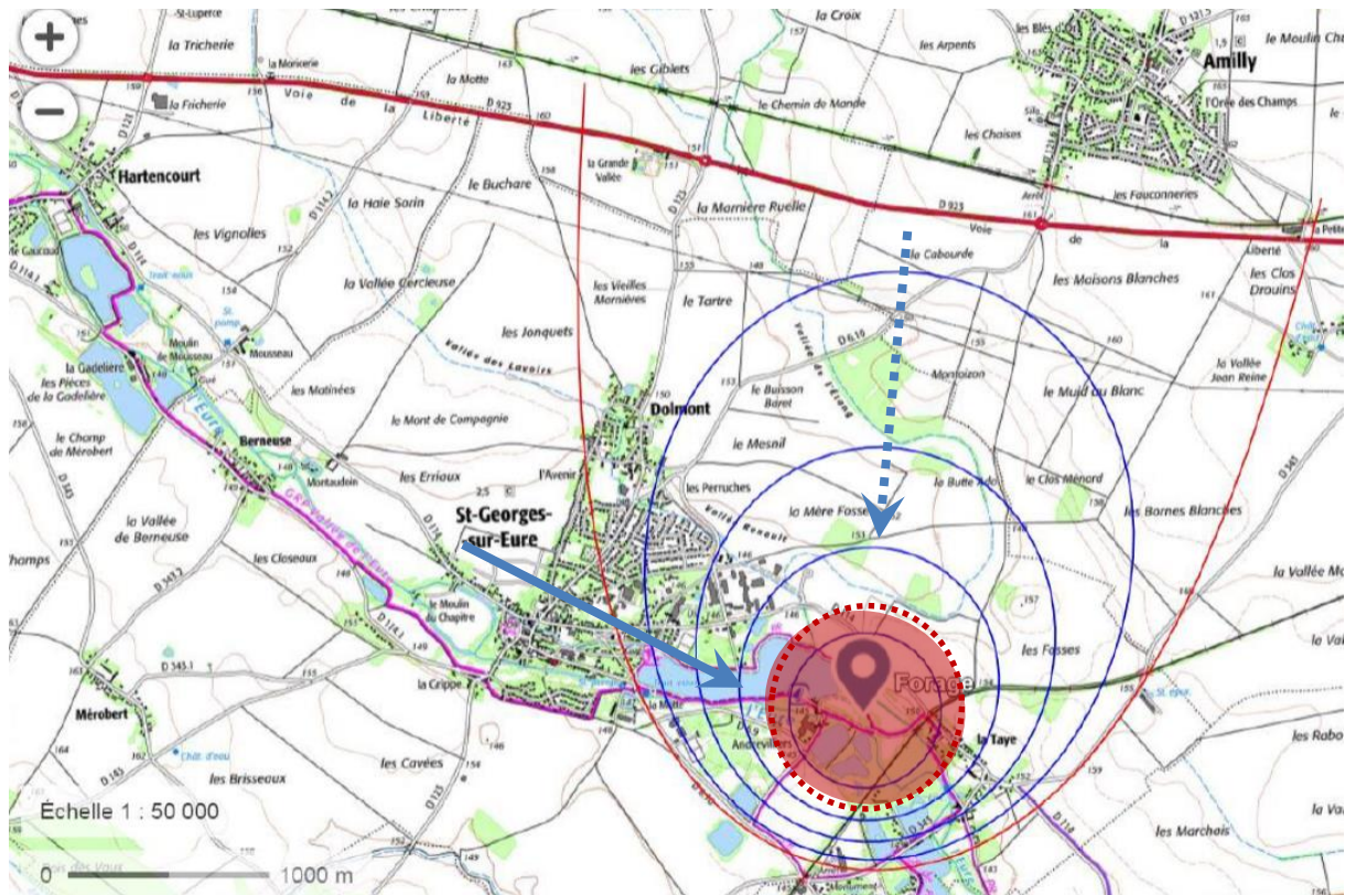
Figure 9. Zone appel et isochrones « 1 mois », « 3 mois », « 6 mois » et « 1 an » autour des forages d'Andrevilliers 1 et 2 en pompage simultané à 400 m 3 /h (Mayer, 2018)
