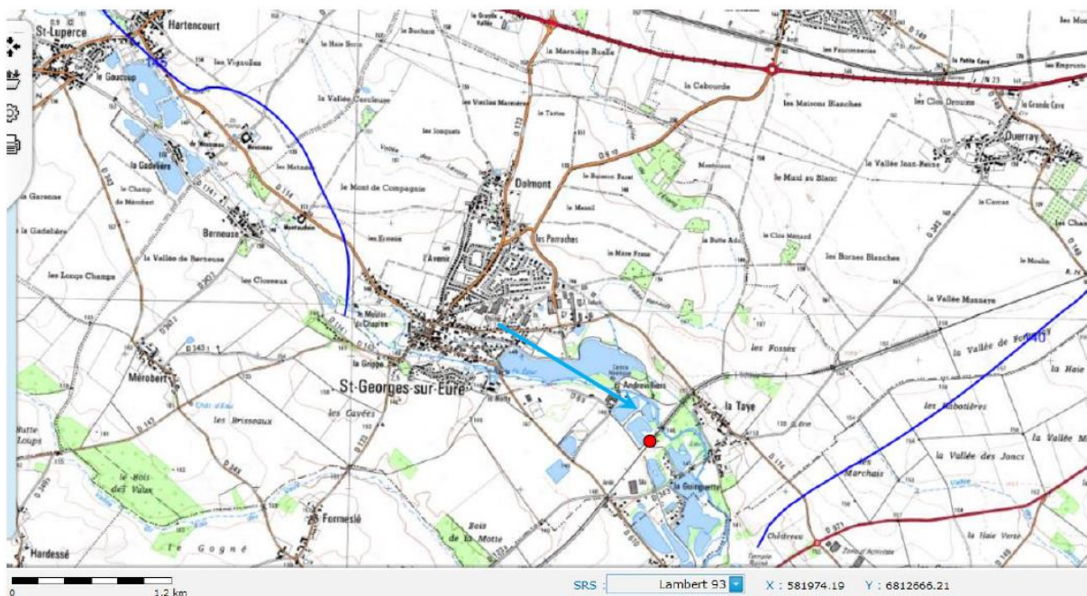
Figure 7. Extrait de la carte piézométrique de la nappe de la craie autour du site d'Andrevilliers marqué par un cercle rouge
