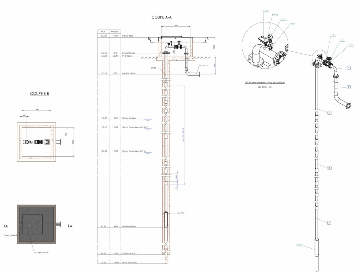
Plan d'équipement de F1
