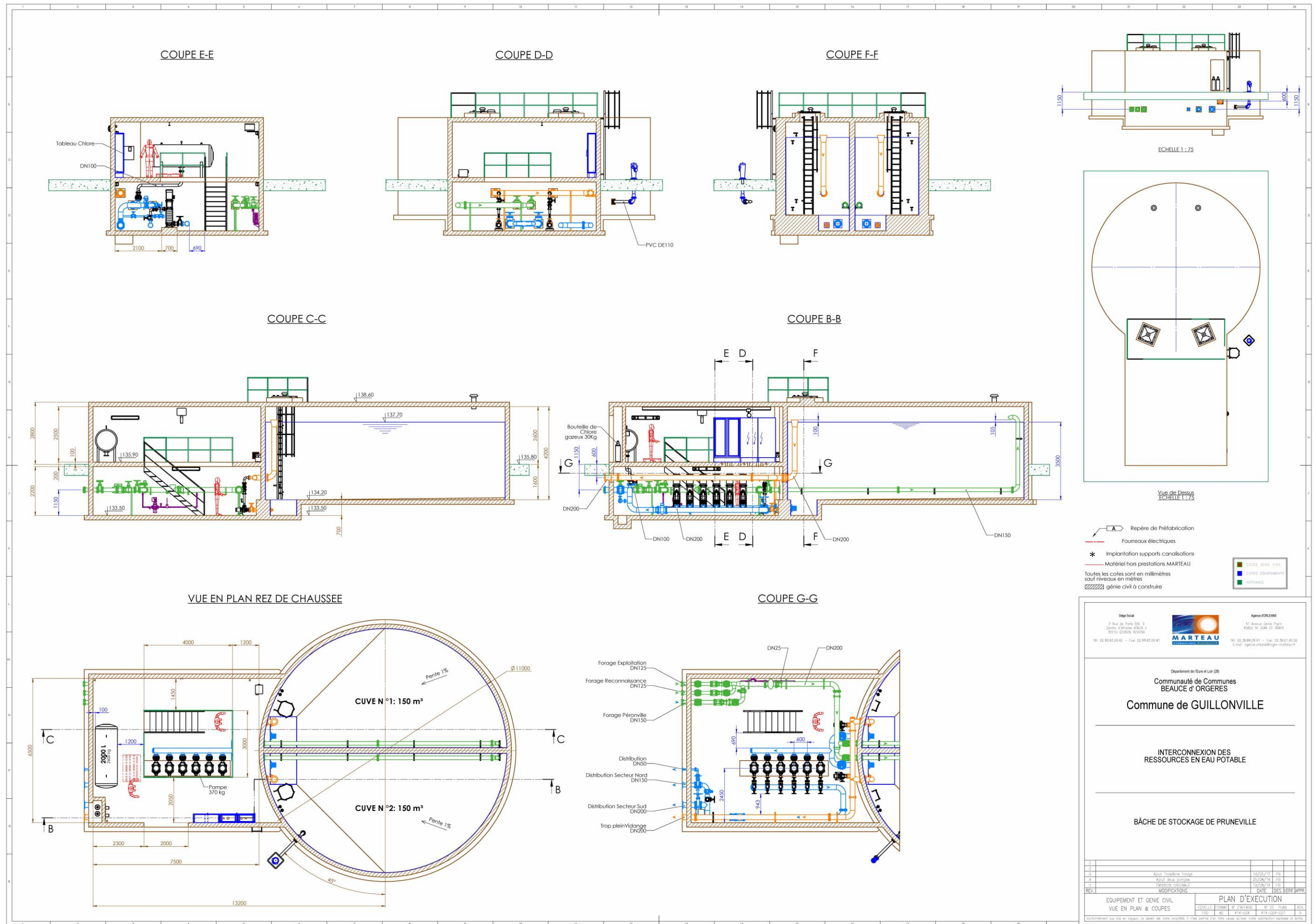
Plan de la station de traitement de l'eau des forages F1 et F2 de Guillonville
