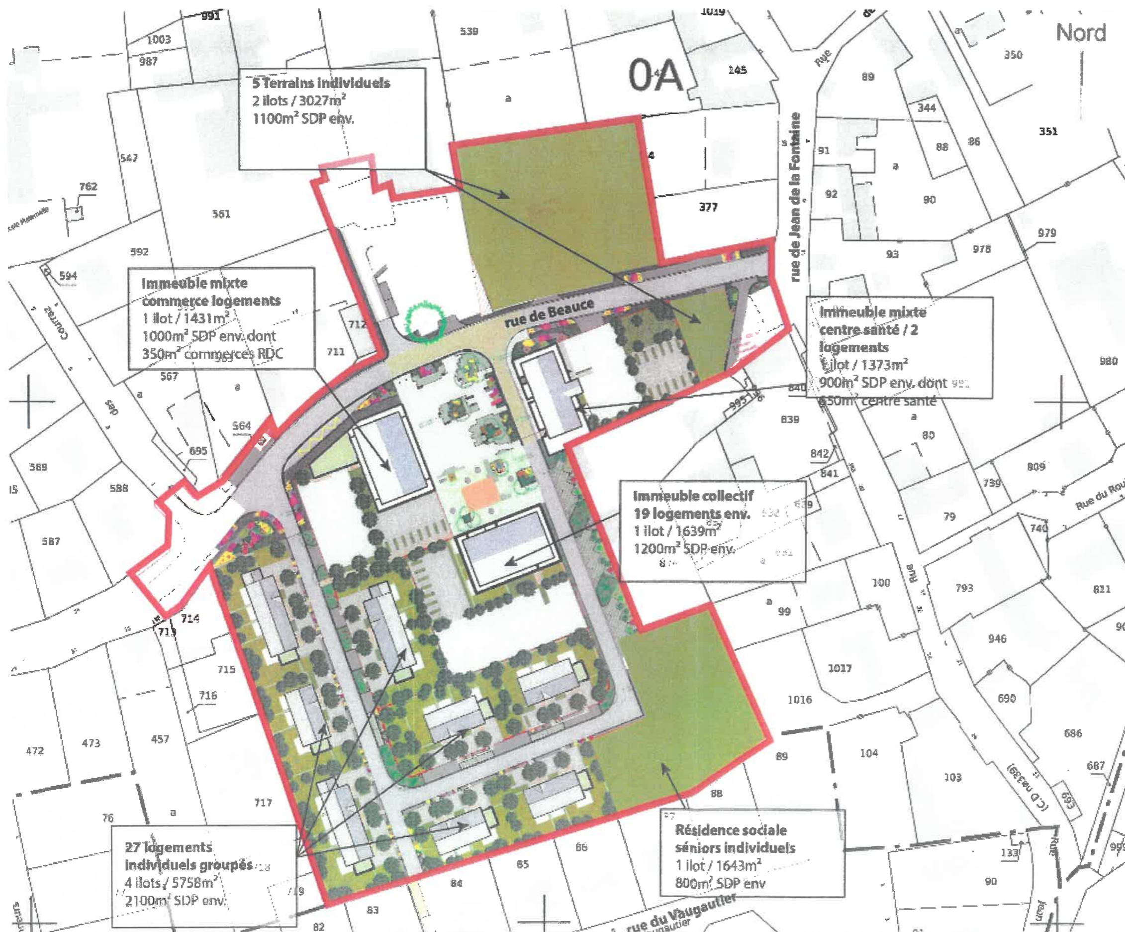
ZAC COEUR DE VILLE - BARJOUVILLE PLAN GENERAL DES TRAVAUX - JAN 2022 ECH 1/1000
